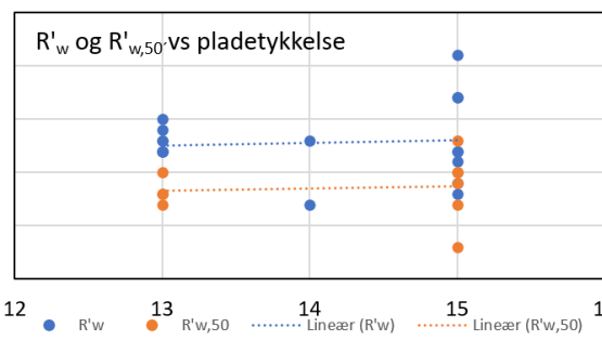
Figur D.5. R'_w øges ikke med pladetykkelsen (mm)
