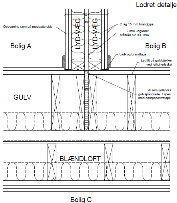
Figur 7.2. Lodret snit mellem rummoduler. Lyd-væg mod gulv i øverste modul, der er opdelt i to boliger. Tegning leveret af Scandibyg A/S.
