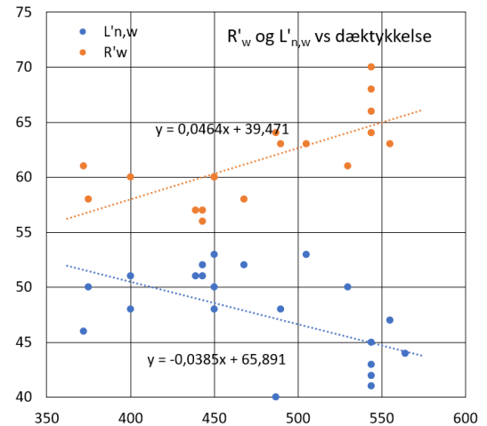
Figur D.2 Relation mellem lyd isolation og dækykkelse i mm.
